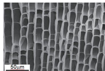
ゲル化凍結法による隔壁構造多孔体 気孔率98%、熱伝導率0.05W/(m·k)
