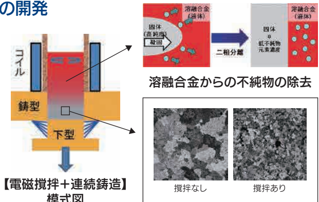
電磁攪拌プロセスによるアルミニウム合金組織の微細化
