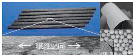
短繊維長CFの配向制御による高性能CFRP化
