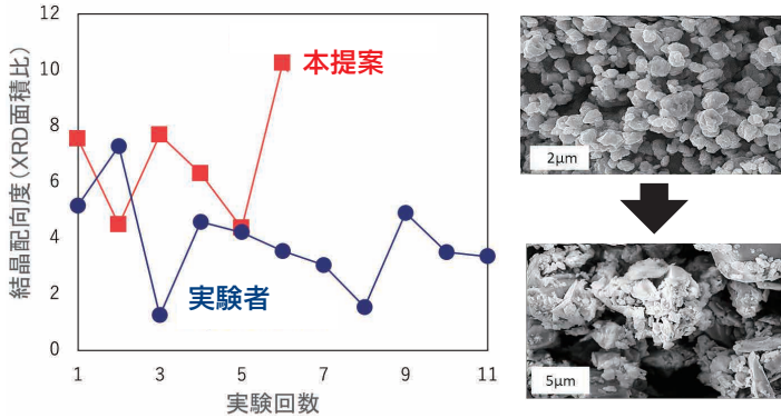
データスクリーニングを併用した ベイズ最適化による高結晶配向度粉末作製
