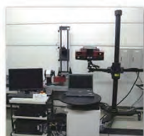
非接触三次元 デジタイザ ATOS III Triple Scan (GOM社)
