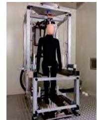
発汗や体表面温度を制御できる発汗サーマルマネキン
