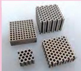
金属3Dプリンタによるタングステンの造形
