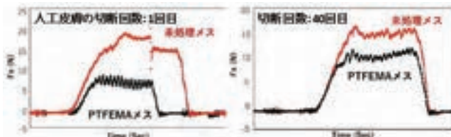
【6軸多関節ロボットによる切れ味試験結果】
