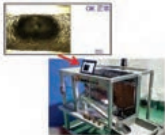
検査装置の外観と判定画面
