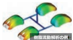
樹脂流動解析の例
