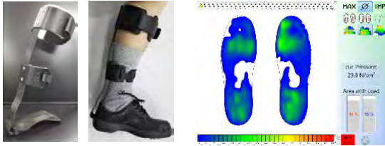
インソール付き下肢装具 (左：外観、右：装着時)
