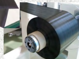
開織技術を用いた炭素繊維薄層プリプレグシート
