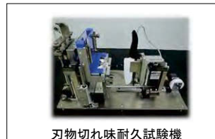
刃物切れ味耐久試験機
